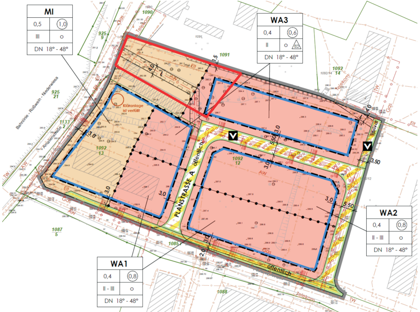
Bebauungsplan Nr. 16. Blau umgrenzt: Baufelder. Rot als ca. Nachtrag: gegenständlicher Bereich
